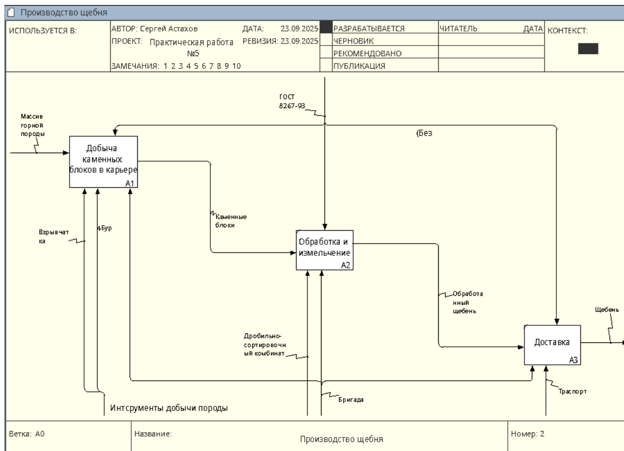
Рисунок 2 — Декомпозиция концептуальной схемы
